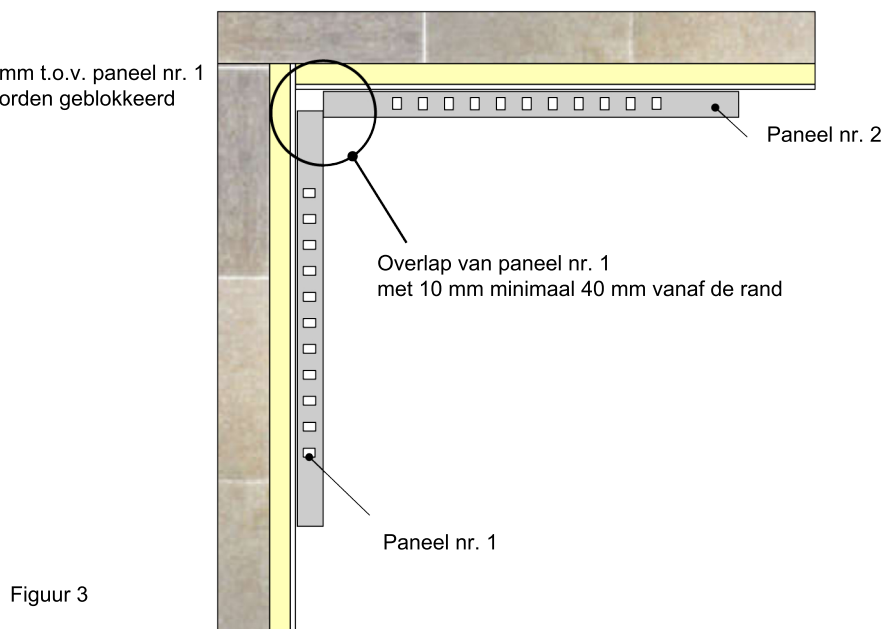
Figuur 3 - Het muurbeschermingspaneel installeren in een hoek met details over de montage van paneel nr. 1
